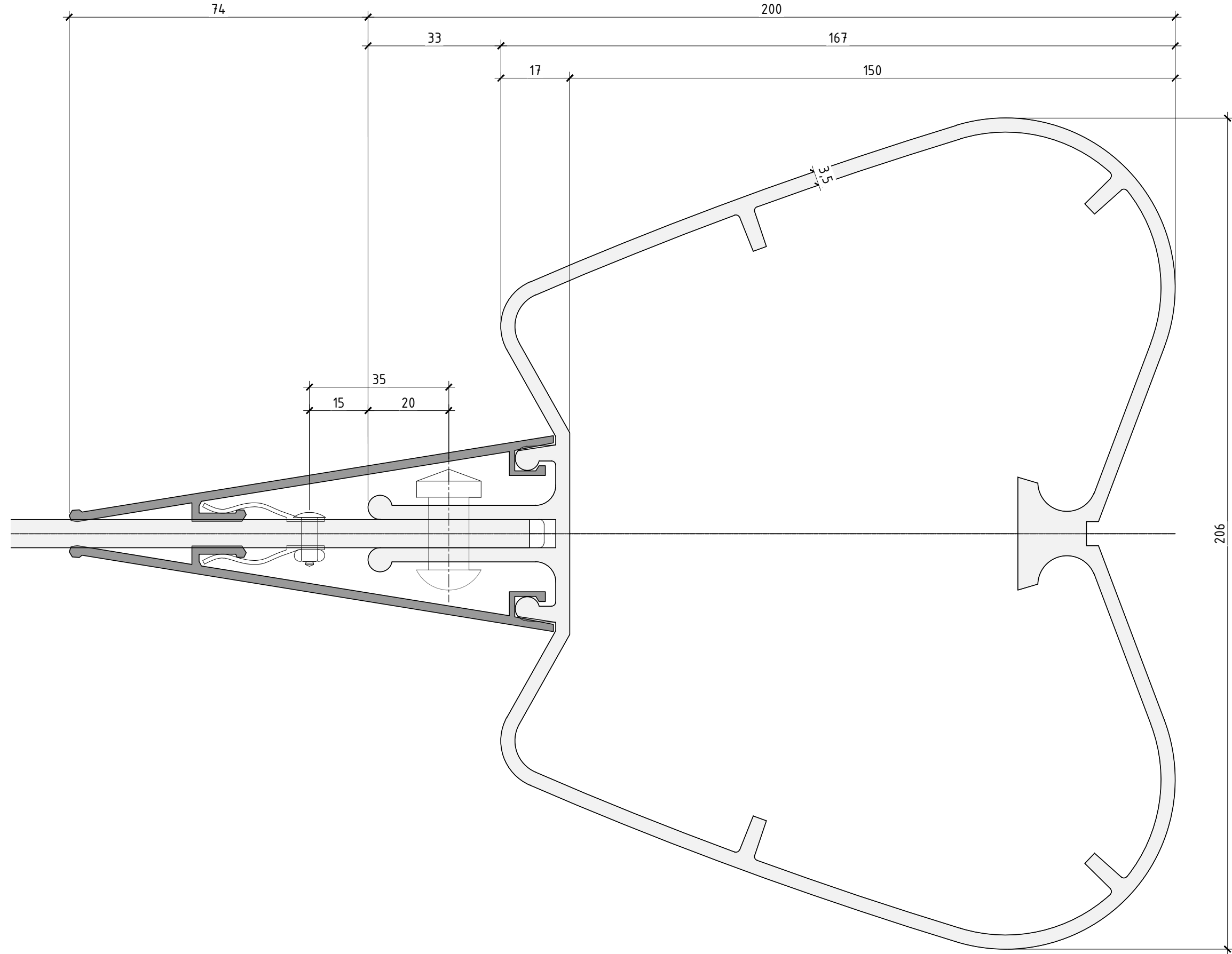
COUPE DE PRINCIPE NOUVELLE COQUE ECH 1:1
