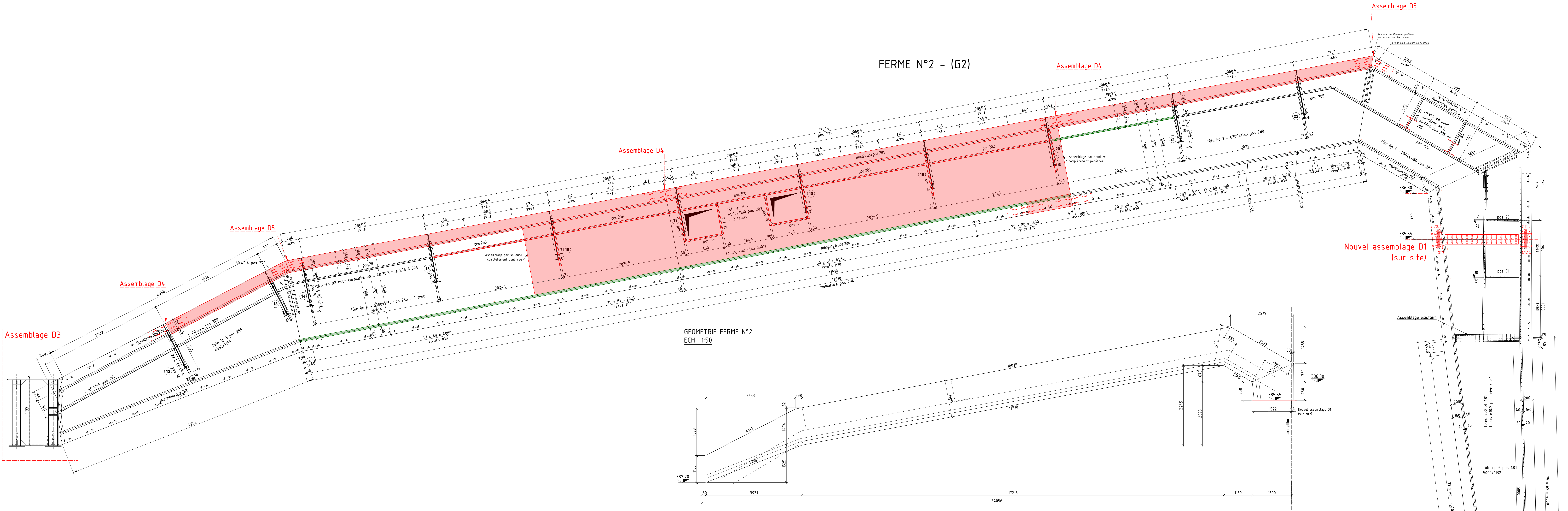
COUPE DE PRINCIPE FERME EXISTANTE ECH 1:1
